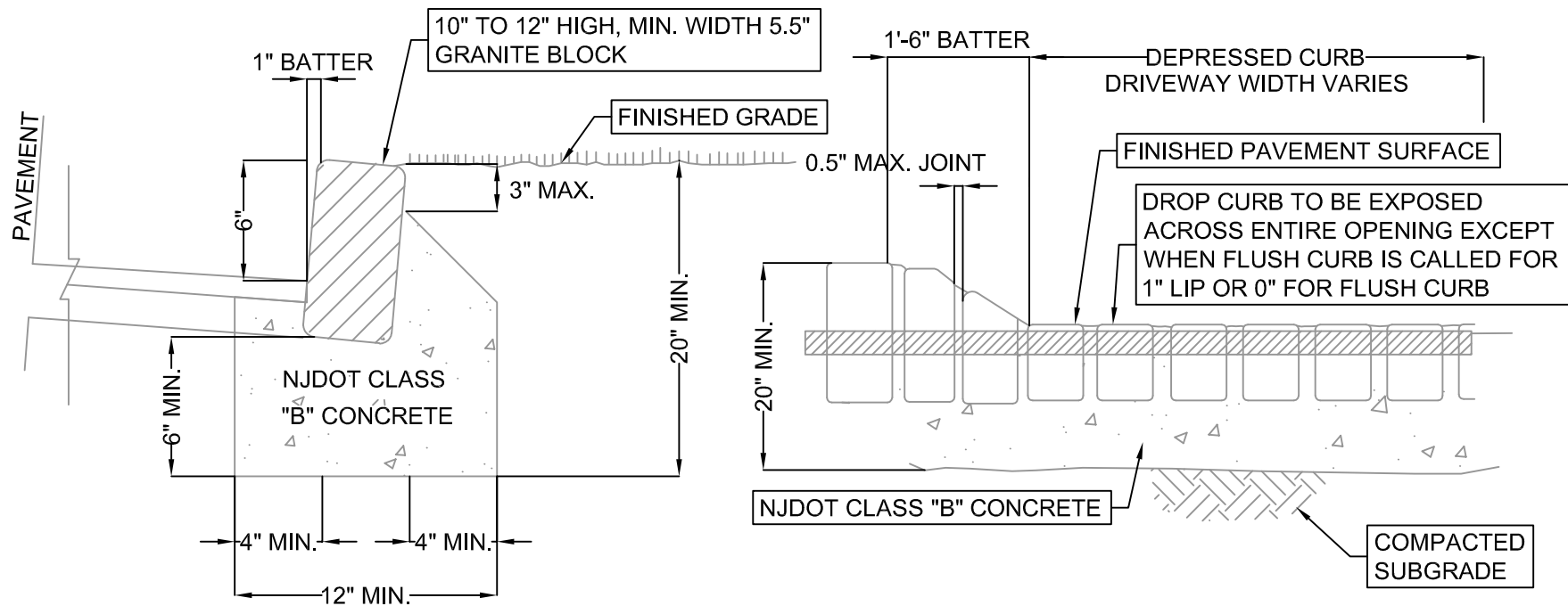
DEPRESSED GRANITE BLOCK CURB N.T.S.
